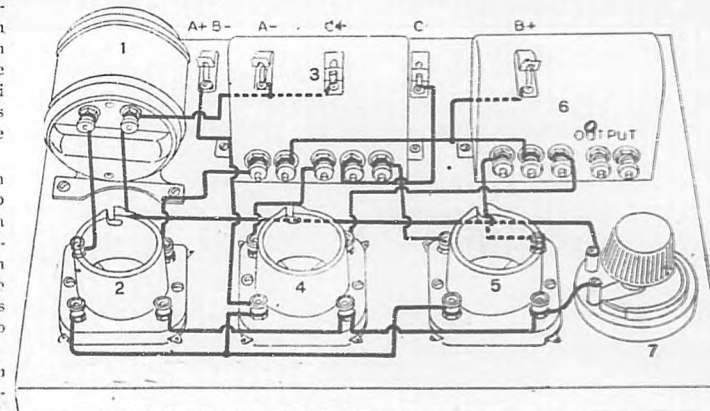
AMPLIFICADOR PUSH-PULL
